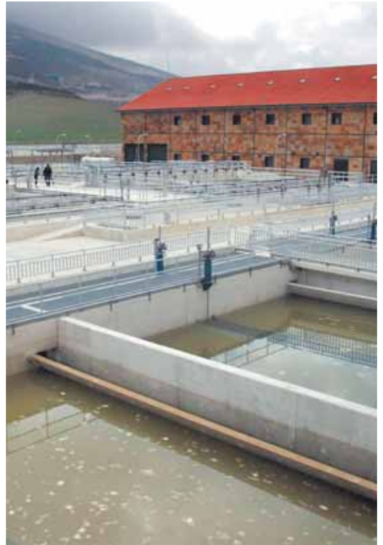
Imagen de la depuradora de Tiebas.
